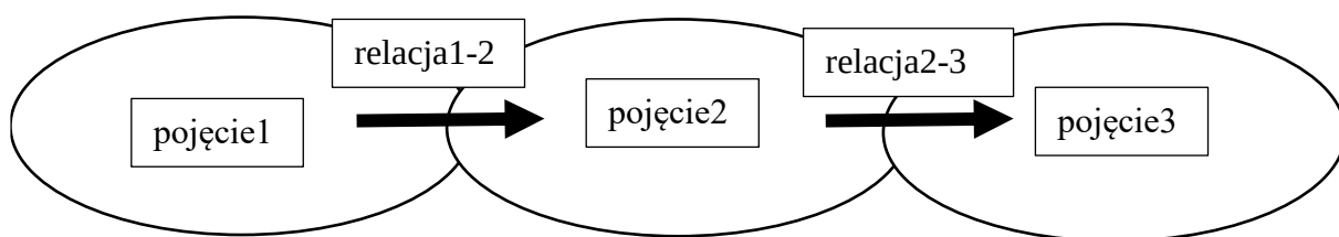
Rysunek 4 Schemat konstruowania dla Cantora.
