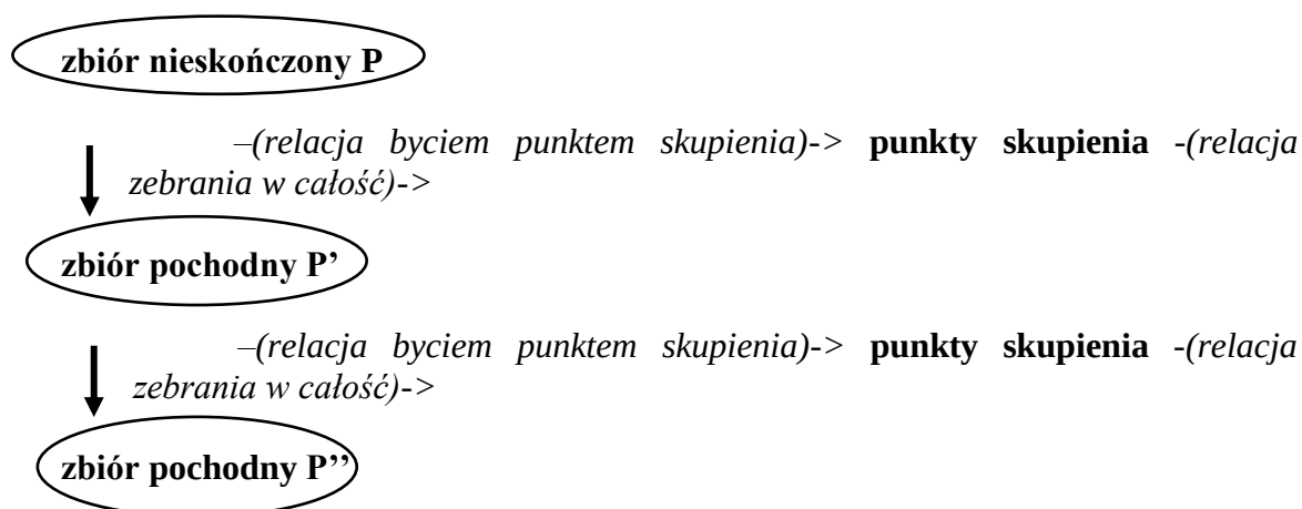
... Rysunek 6 Schemat konstrukcji zbiorów pochodnych przez Cantora.
