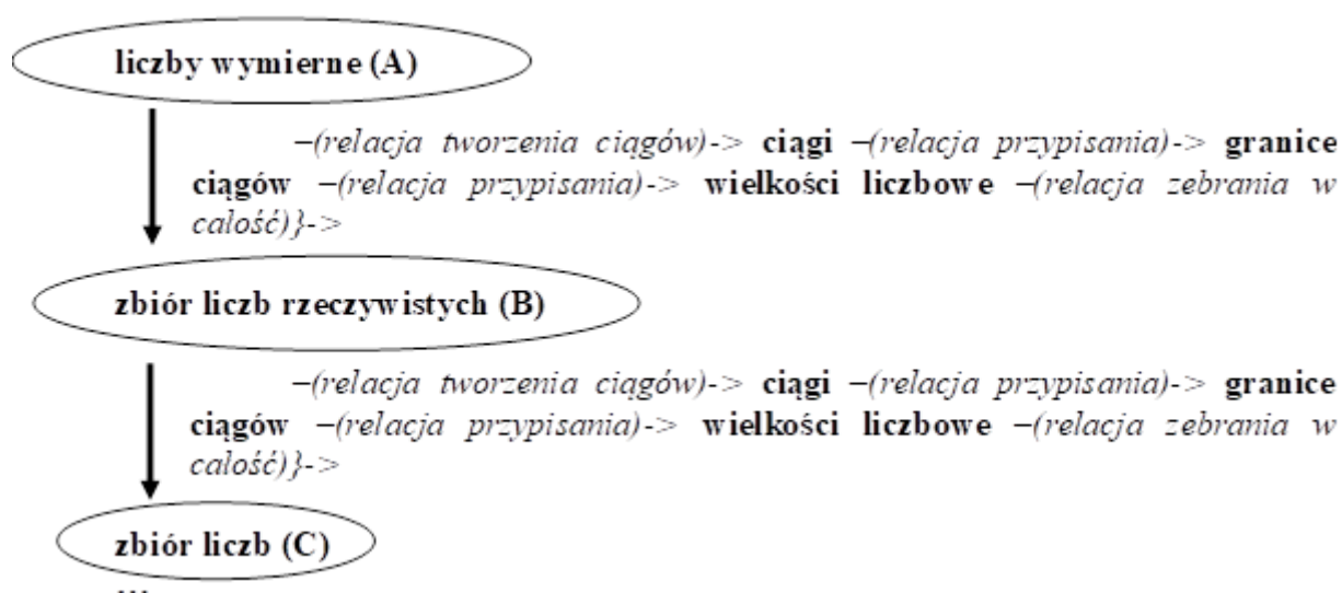
Rysunek 5 Schemat konstrukcji liczb rzeczywistych przez Cantora.
